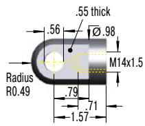
A14 Eye
