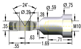
E10 Swivel Eye DIN 648
