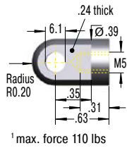
A5-VA Eye
